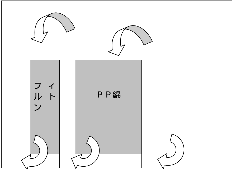
断面図
